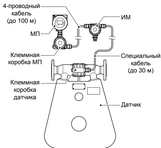
Рис. 7. Раздельно-выносное исполнение
