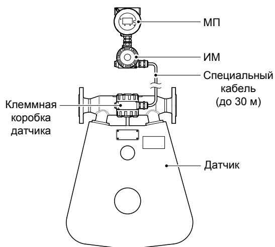
Рис. 5. Раздельное исполнение
