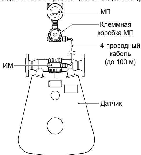
Рис. 6. Выносное исполнение
