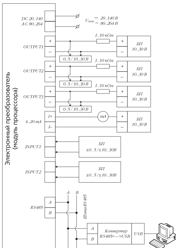
Рис. 12. Схема подключения ЭП расходомера к внешним устройствам.
